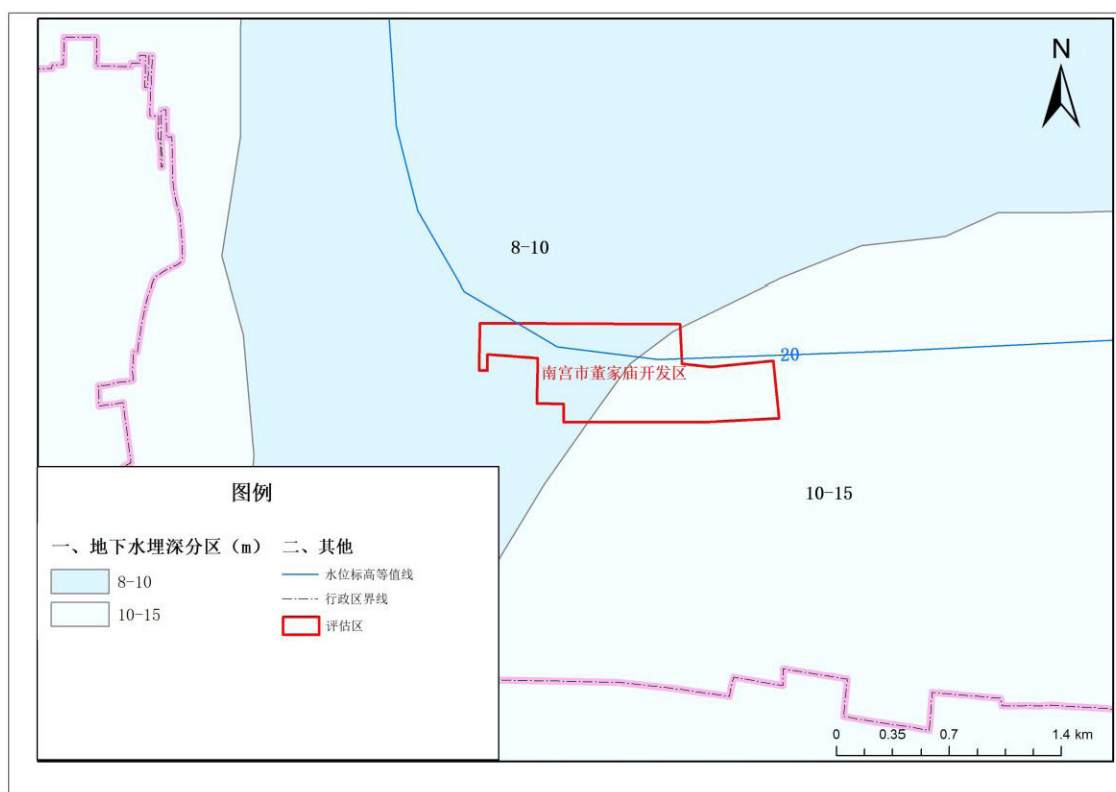
图2-5 2020年6月浅层地下水及标高等值线图
