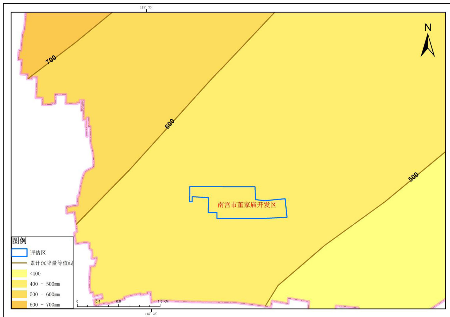
图3-1 1978-2018年底累计地面沉降图
