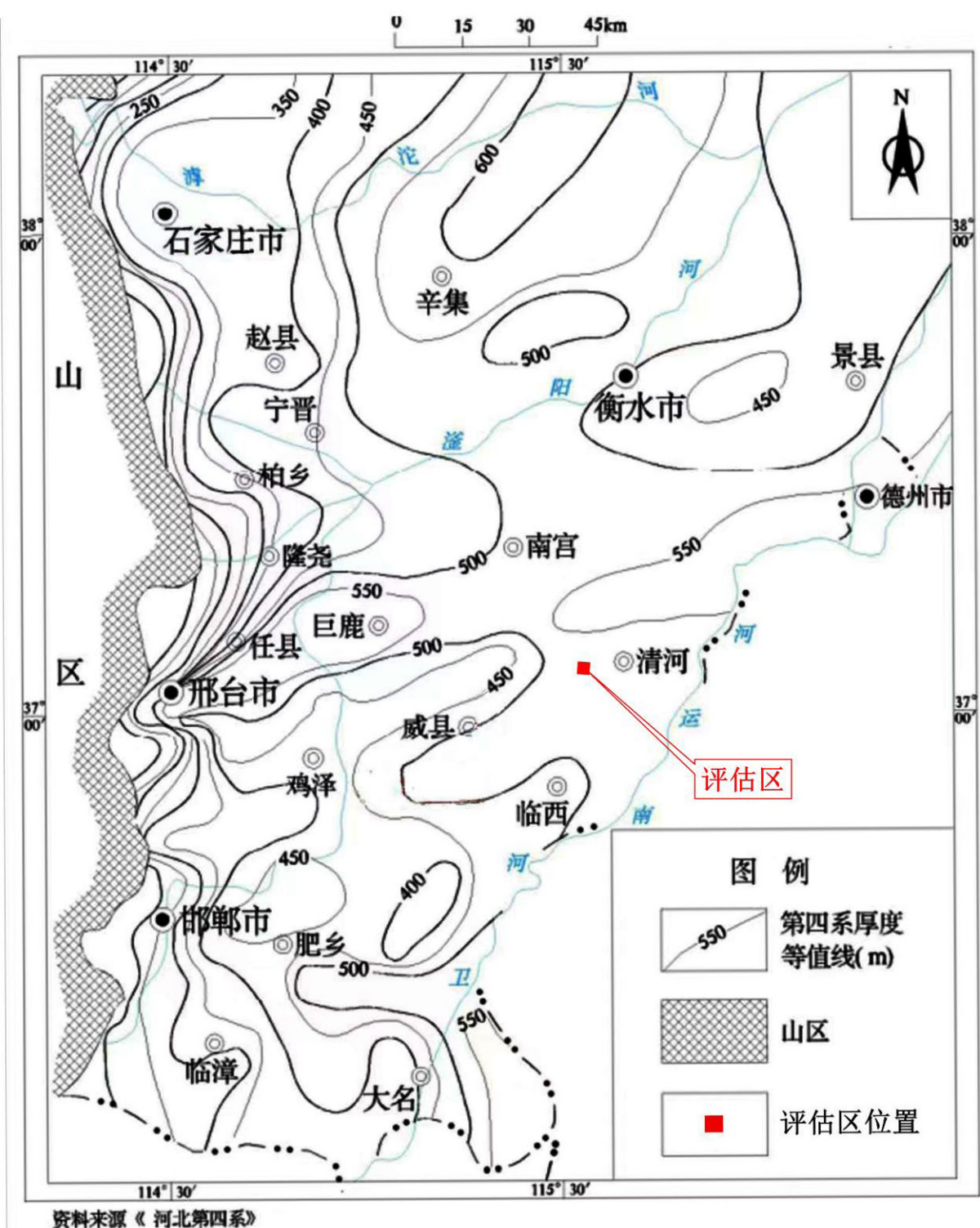
图2-2第四系厚度等值图
