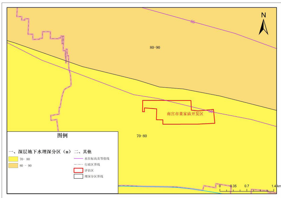
图2-6 2020年6月深层地下水及标高等值线图
